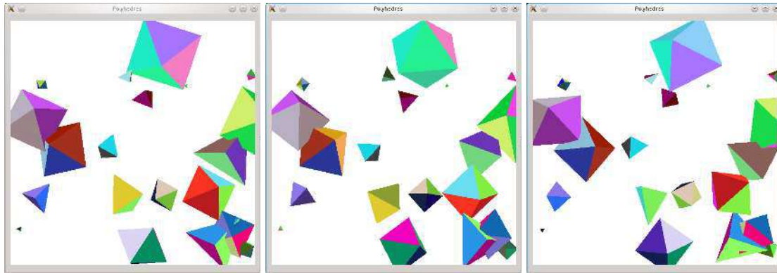
FIGURE B.2 – Des tétraèdres et octaèdres en rotation dans l’espace. Aucun traitement particulier n’est fait pour les solides qui s’intersectent.
