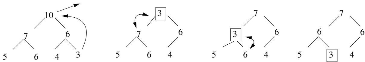
FIGURE 14.2 – Fonction pop dans la file de priorité
