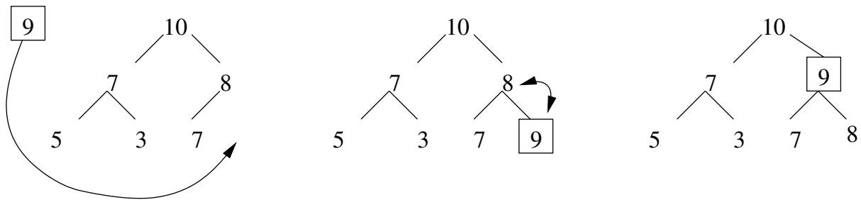
FIGURE 14.1 – Fonction push dans la file de priorité
