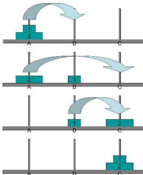
FIGURE B.10 – Solution du problème pour N=2
