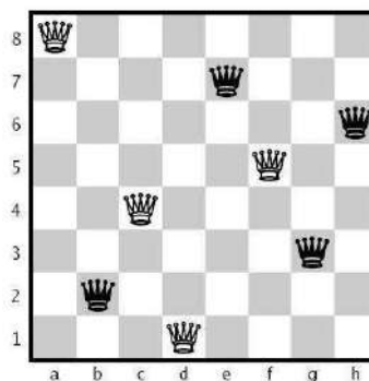
FIGURE B.13 – Une solution du problème des huit dames
