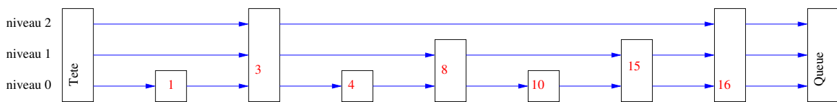
FIGURE B.11 – Une liste avec sauts. Les valeurs sont triées. Des raccourcis existent aux niveaux 1 et 2 pour une recherche plus rapide.
