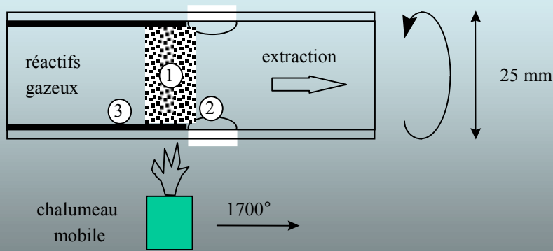
Dépôt de la gaine
