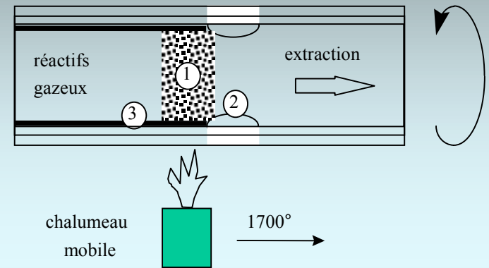
Dépôt du coeur
