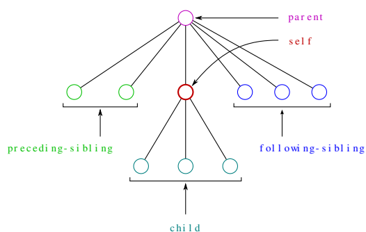
Figure 6.2. Nœuds proches
