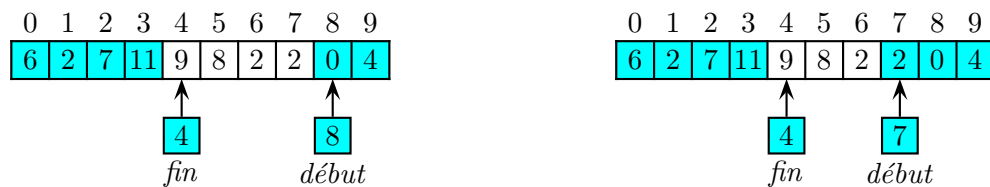
FIG. 4.14 – Suppression dans la file.
