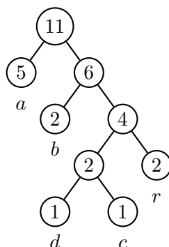
FIG. 5.28 – L'arbre après la dernière fusion.
