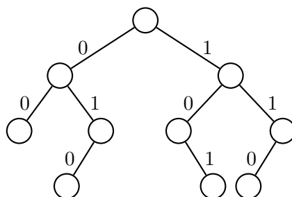
FIG. 5.22 – Le code des feuilles est \{00, 010, 101, 110\} .
