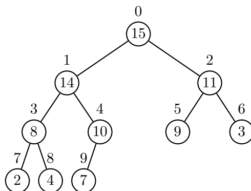
FIG. 4.19 – Le tas de la figure 4.18 après suppression de 16.
