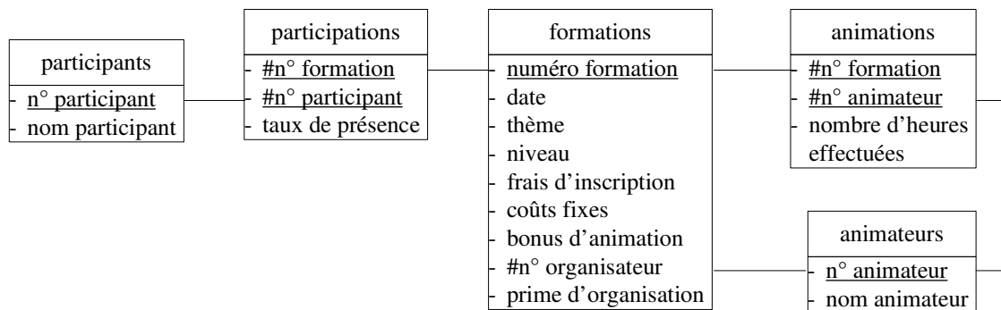
FIG. 7 – Schéma relationnel qui possède un cycle
